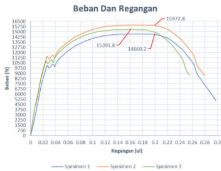
Gambar 6. Grafik Beban – Regangan
