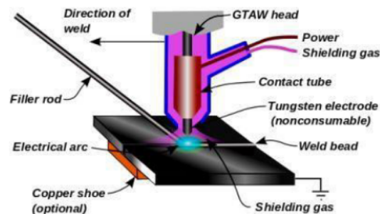
Gambar 1. Mekanisme Las TIG
