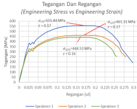
Gambar 5. Grafik Tegangan Tarik – Regangan
