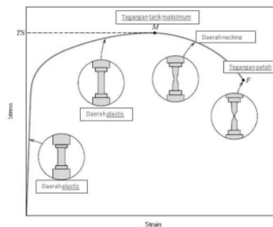
Gambar 2. Kurva Tegangan Regangan
