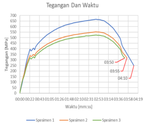
Gambar 4. Grafik Tegangan Tarik - Waktu Patahan Spesimen
